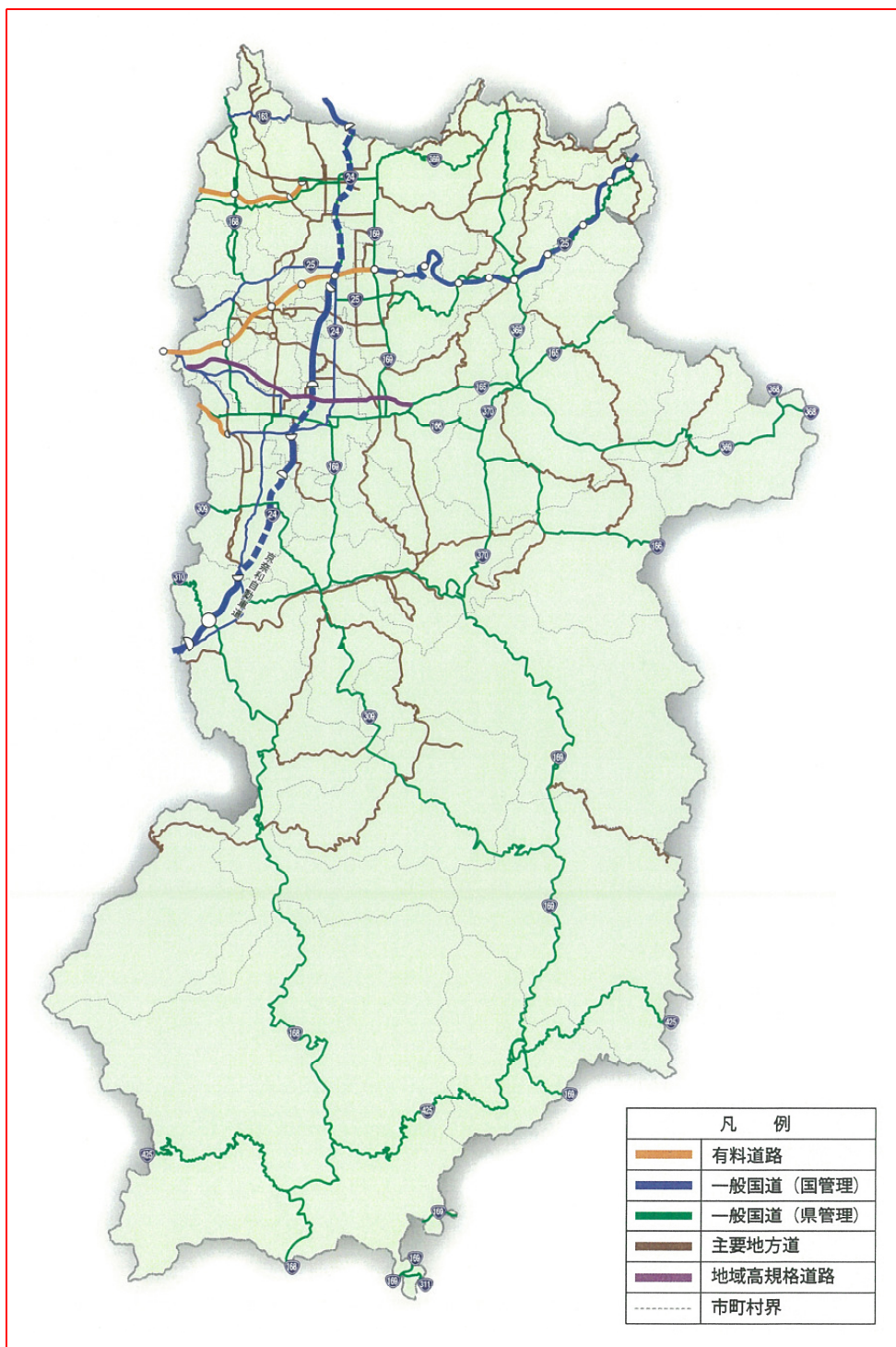
図5 奈良県の幹線道路網（平成26年4月現在）
