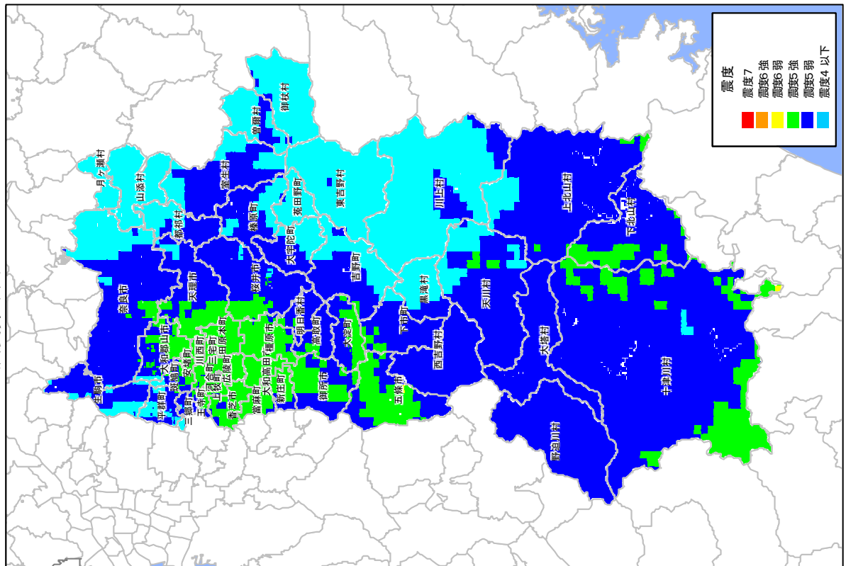
震度分布図
