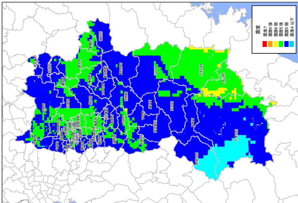
震度分布図
