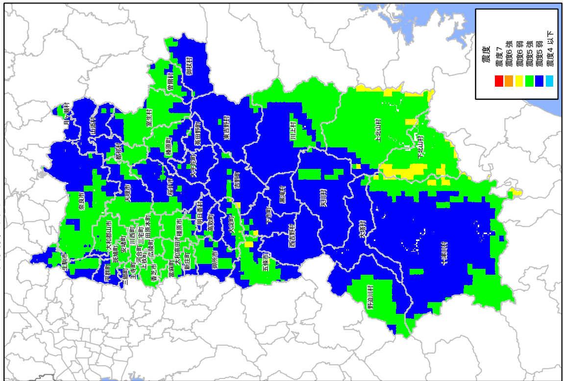
震度分布図
