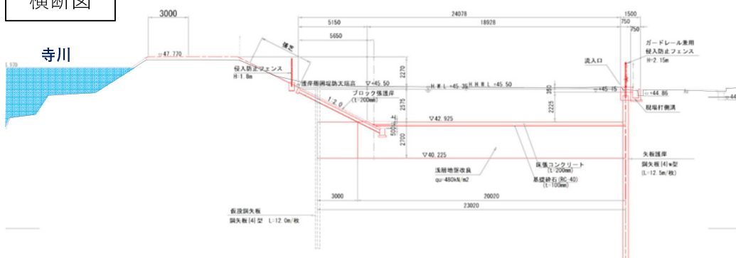
横断面図
