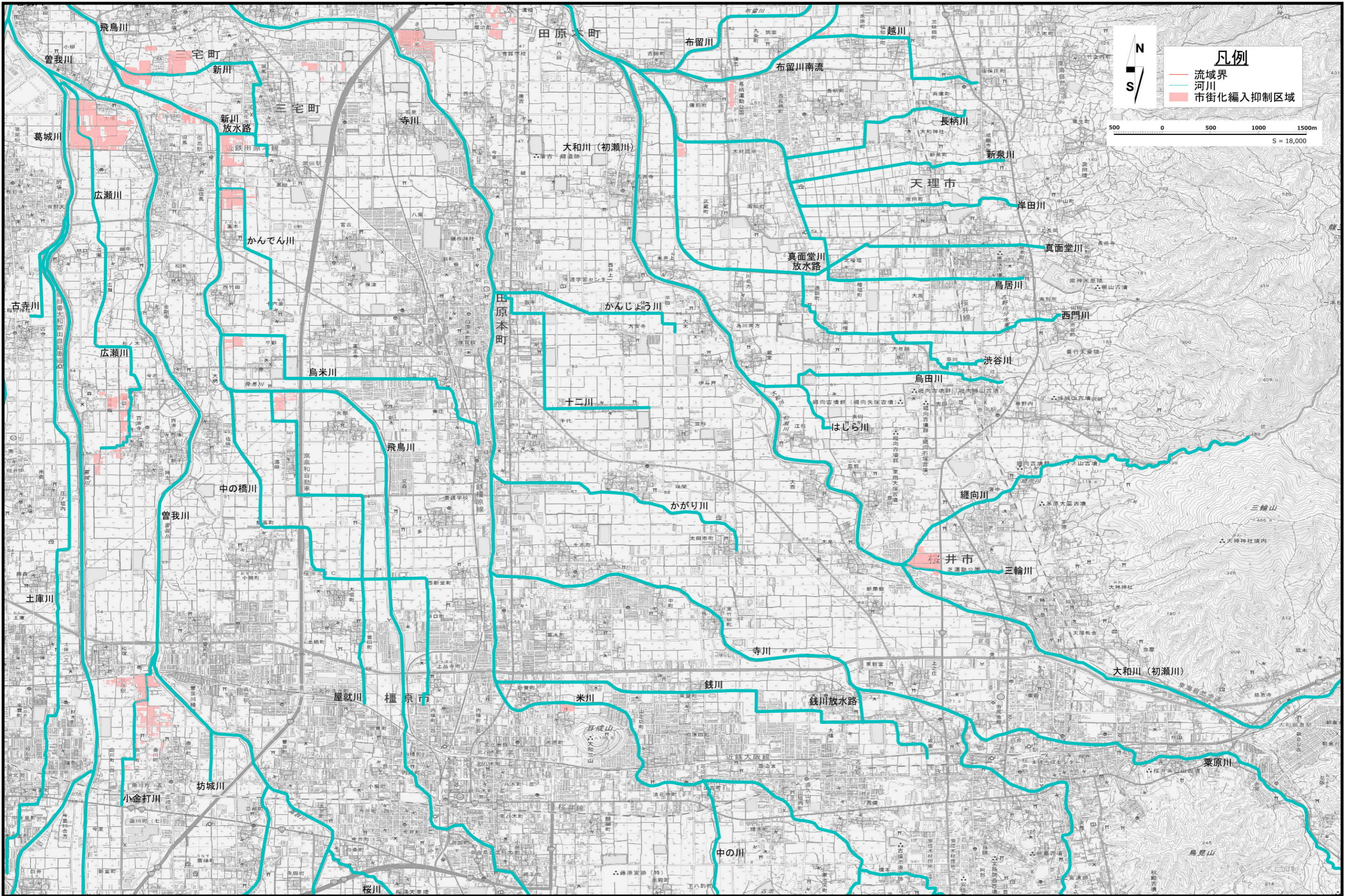
大和川流域 市街化編入抑制区域図 (図面番号⑨)
