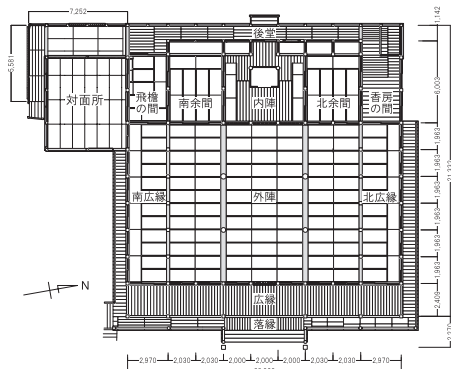
本堂 平面図
