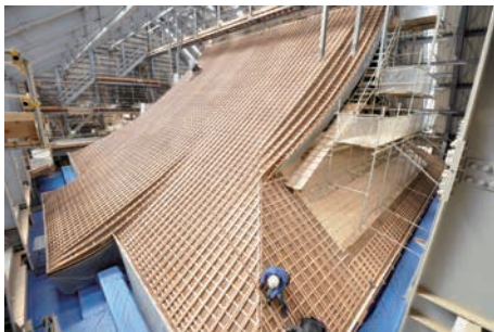
瓦棧施工中
