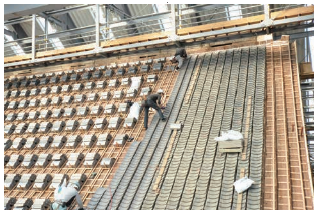
屋根工事（棧木に平瓦をのせる）
