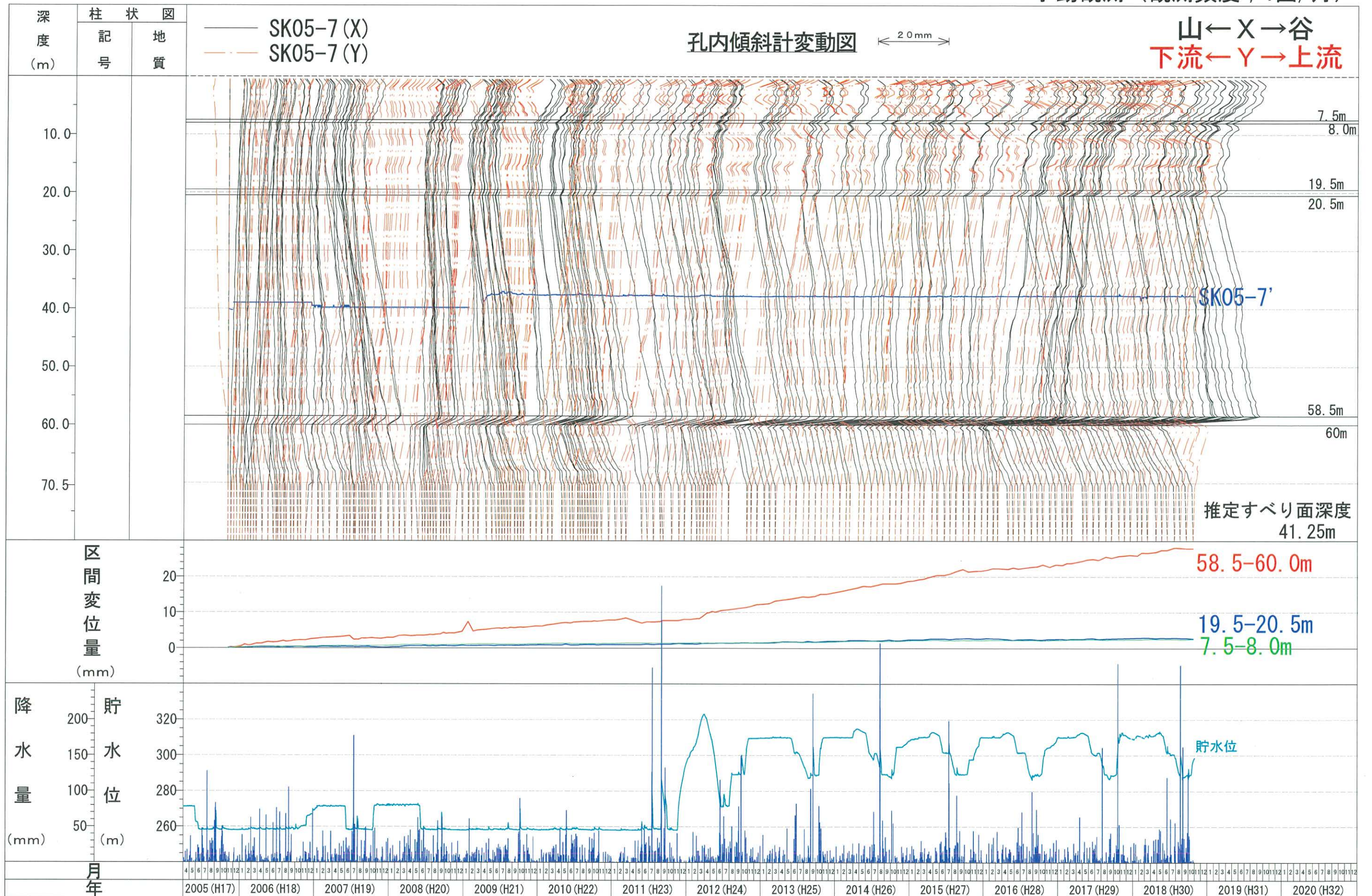
迫地区孔内傾斜計SK05-7変動図
