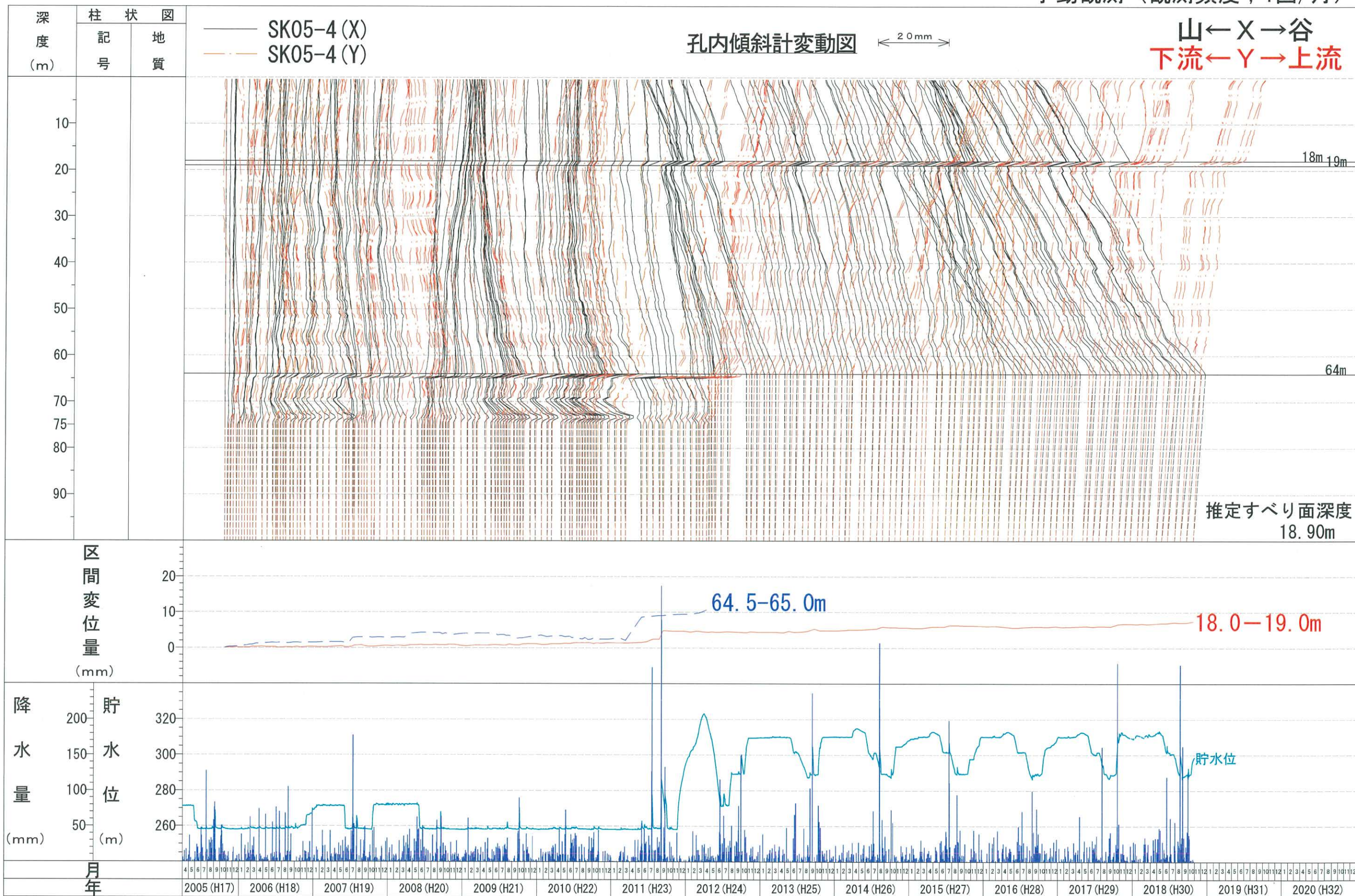
迫地区孔内傾斜計SK05-4変動図
