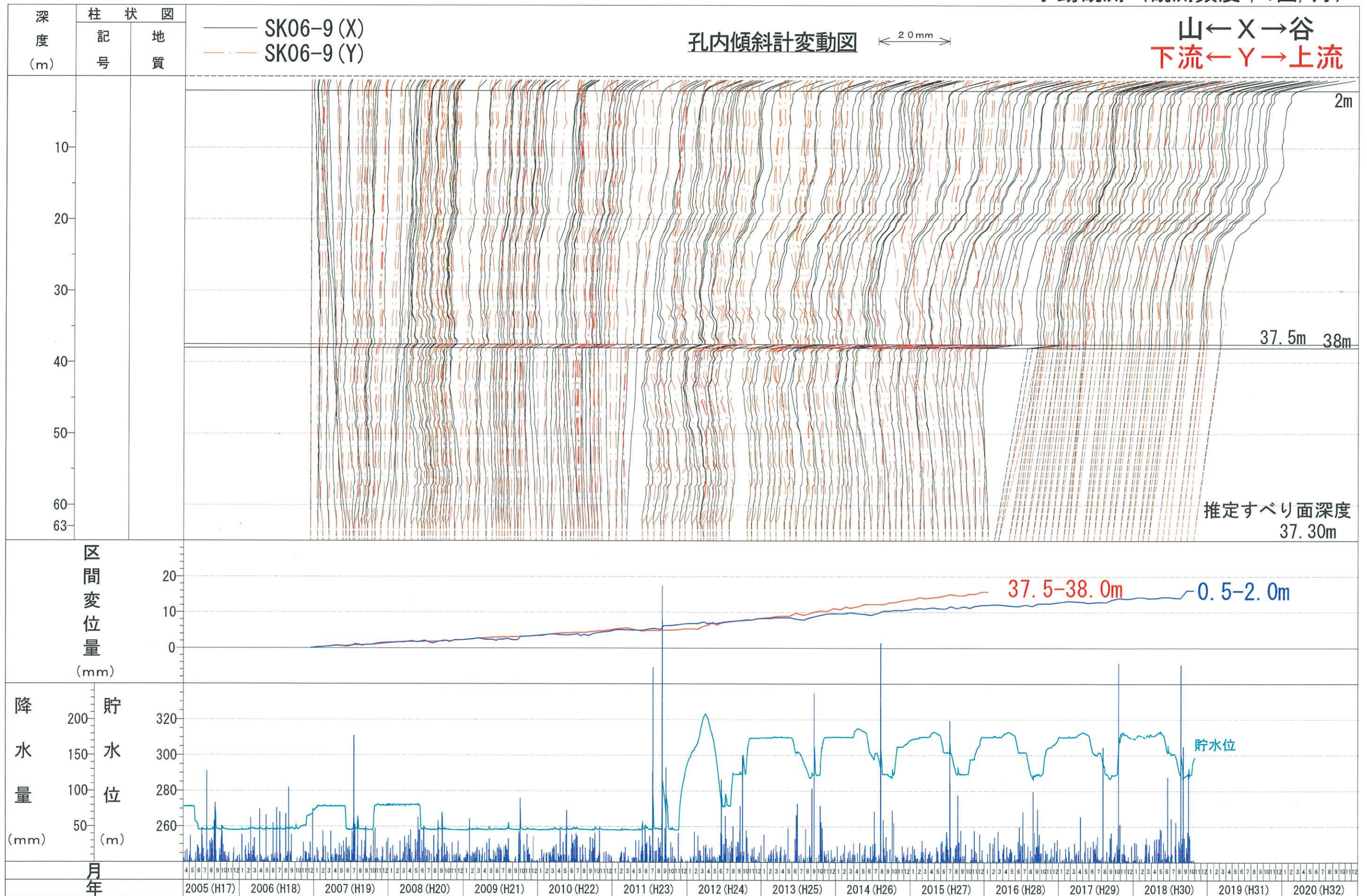
迫地区孔内傾斜計SK06-9変動図
