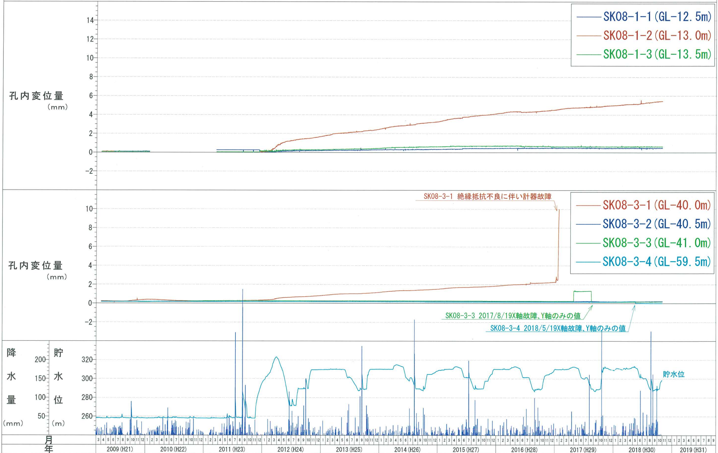
迫地区SK13ブロック孔内傾斜計変動図
