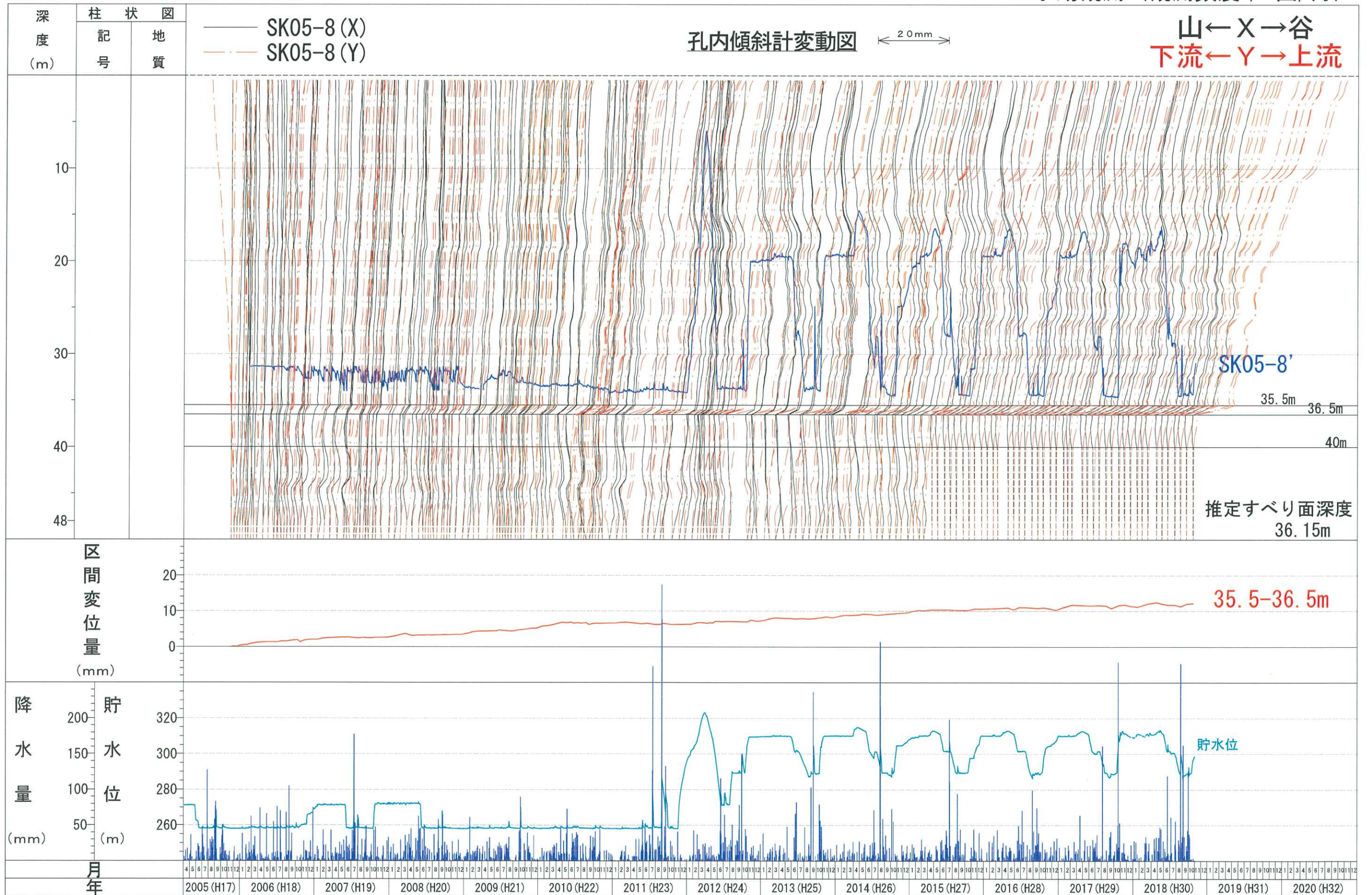
迫地区孔内傾斜計SK05-8変動図
