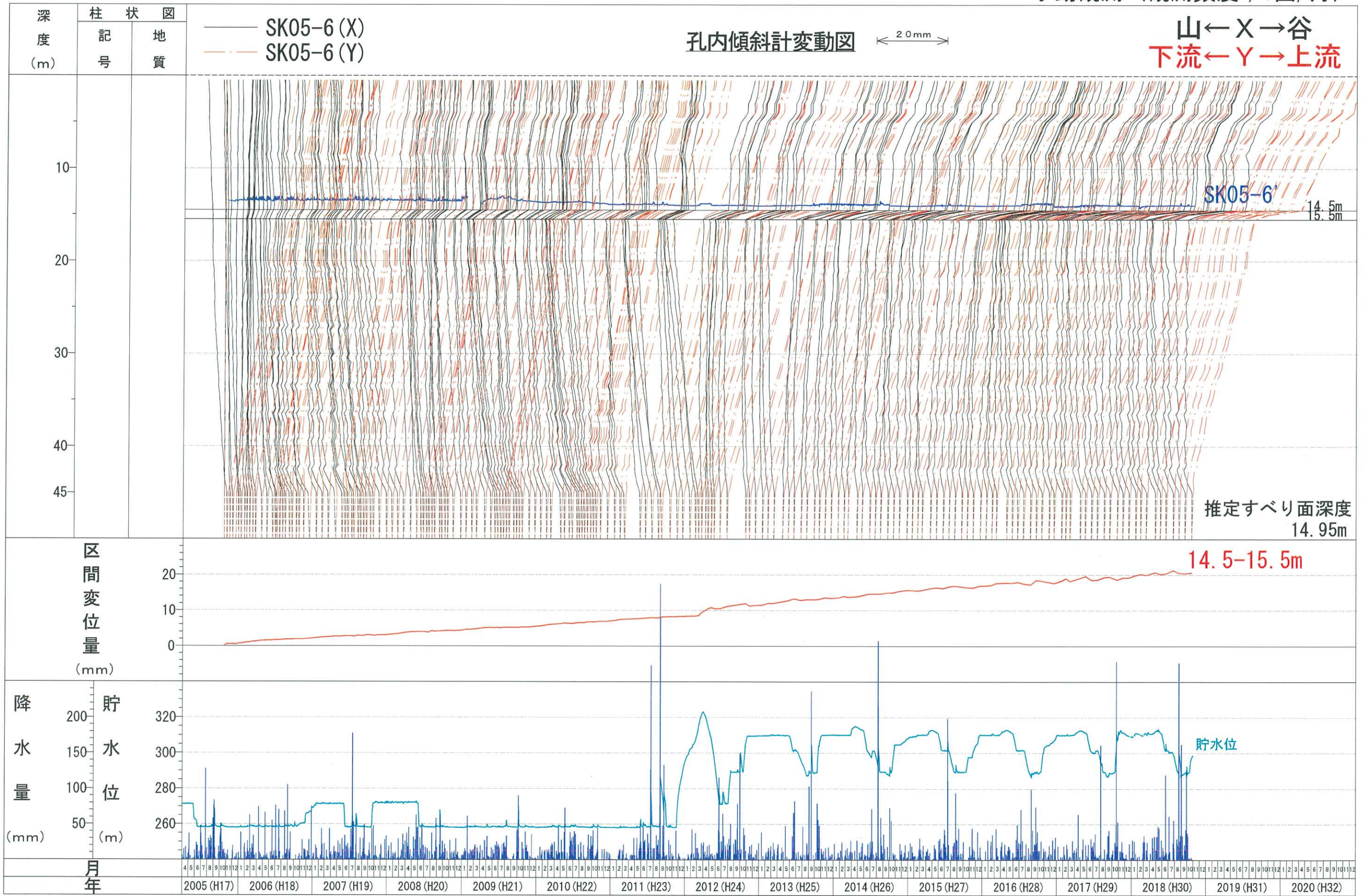
迫地区孔内傾斜計SK05-6変動図
