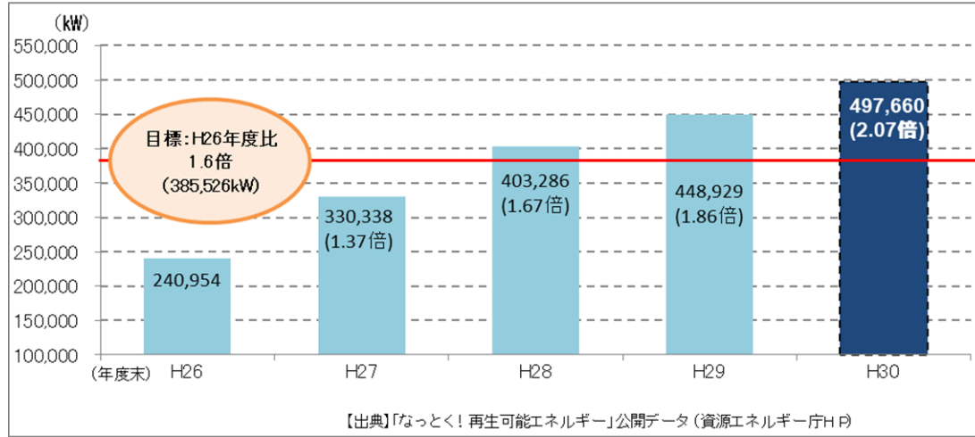
再生可能エネルギーの導入量（設備容量）
