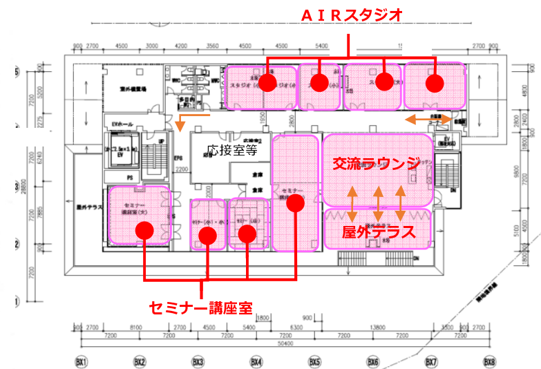
2階平面図
