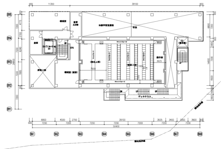
中2階平面図
