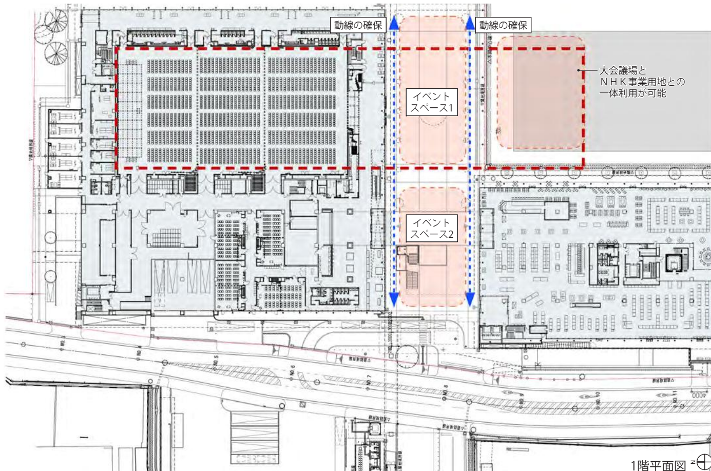
1階平面図
