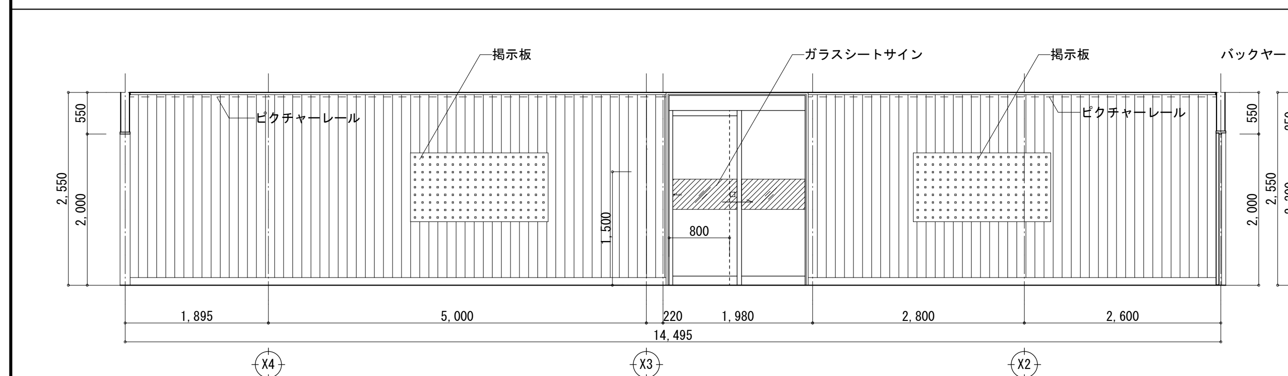
廊下 C面
