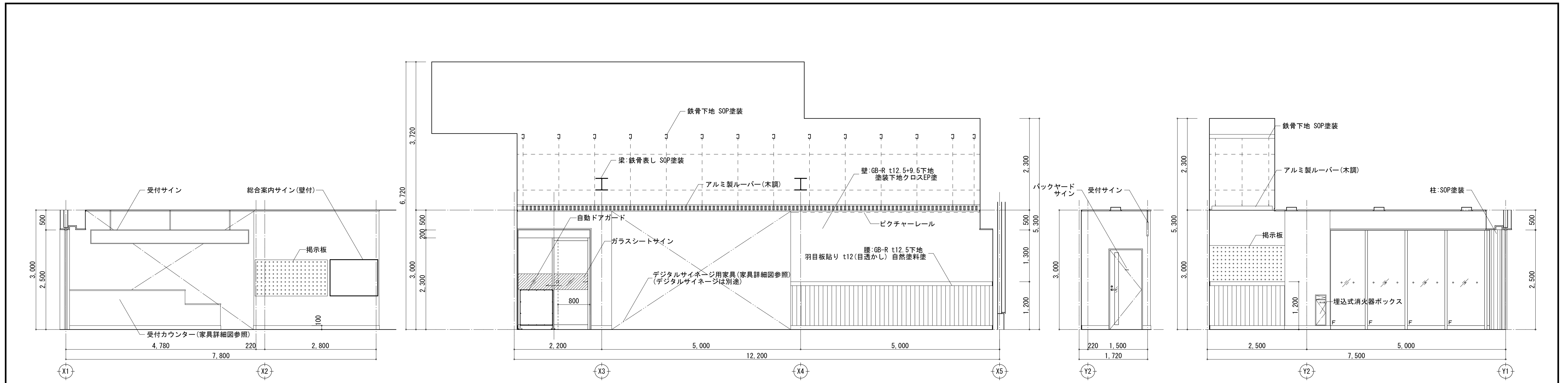
観光案内スペース・キッズスペース・休憩スペース
