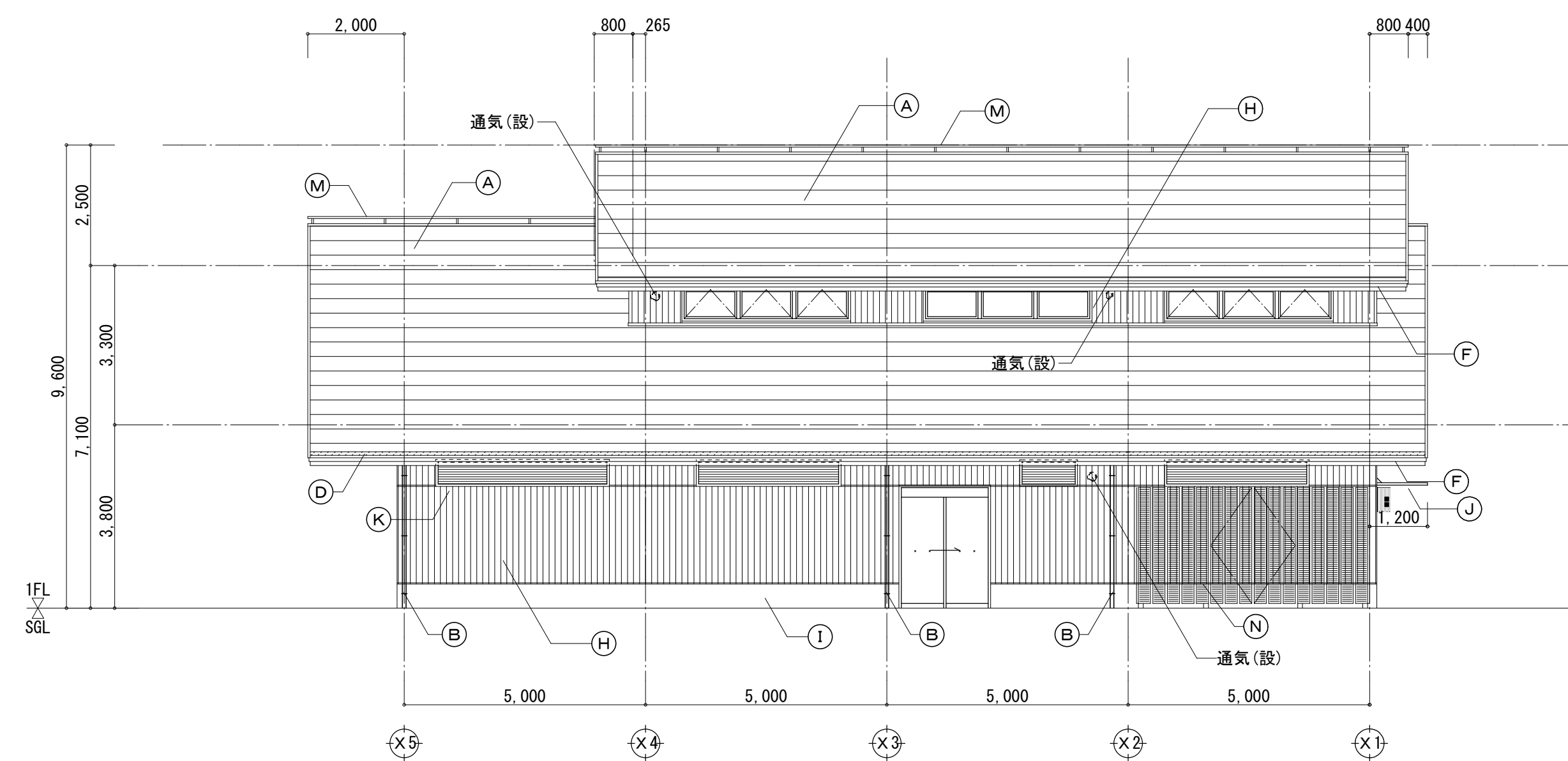
北側立面図
