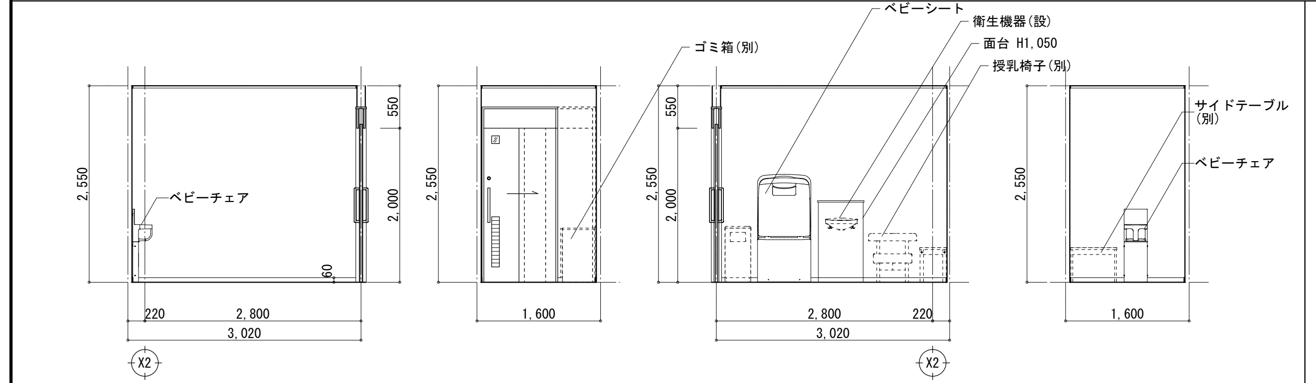
授乳室2~3 A面 B面 C面 D面 倉庫1 A面 B面 C面 D面
