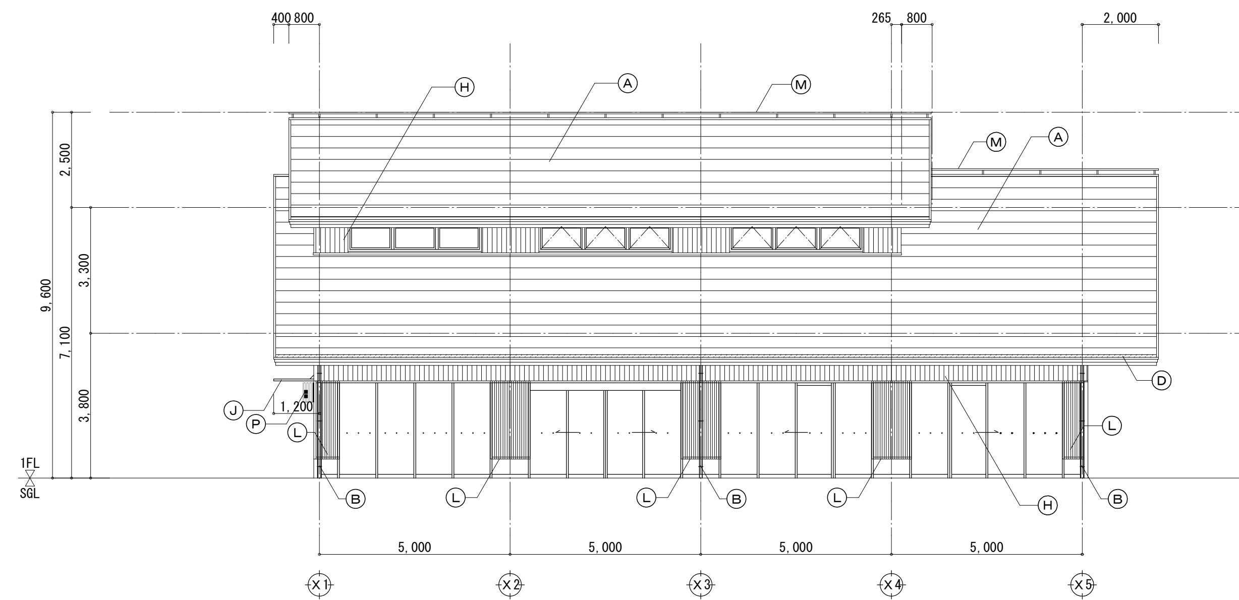
南側立面図
