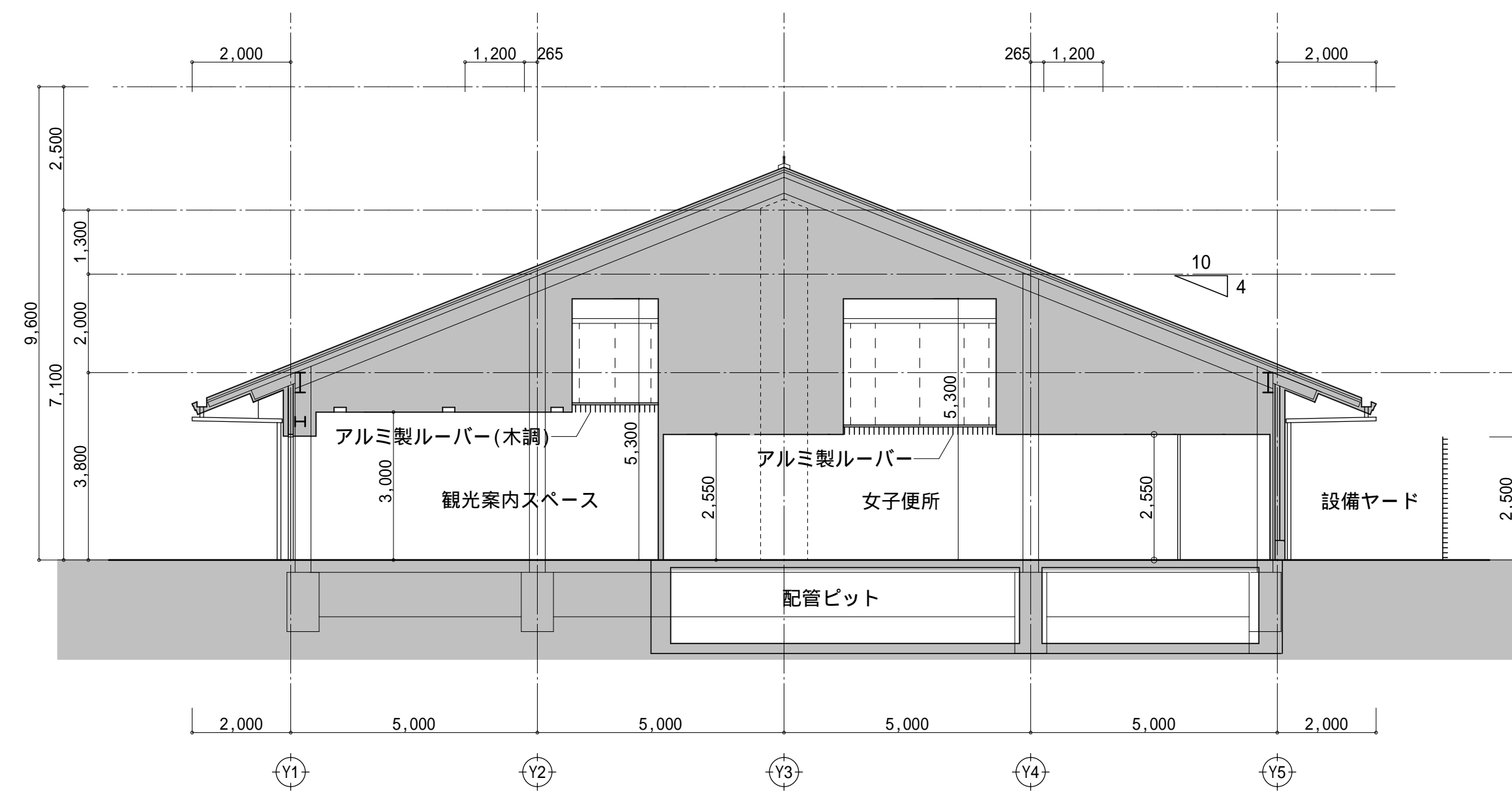
X 方向断面図 2
