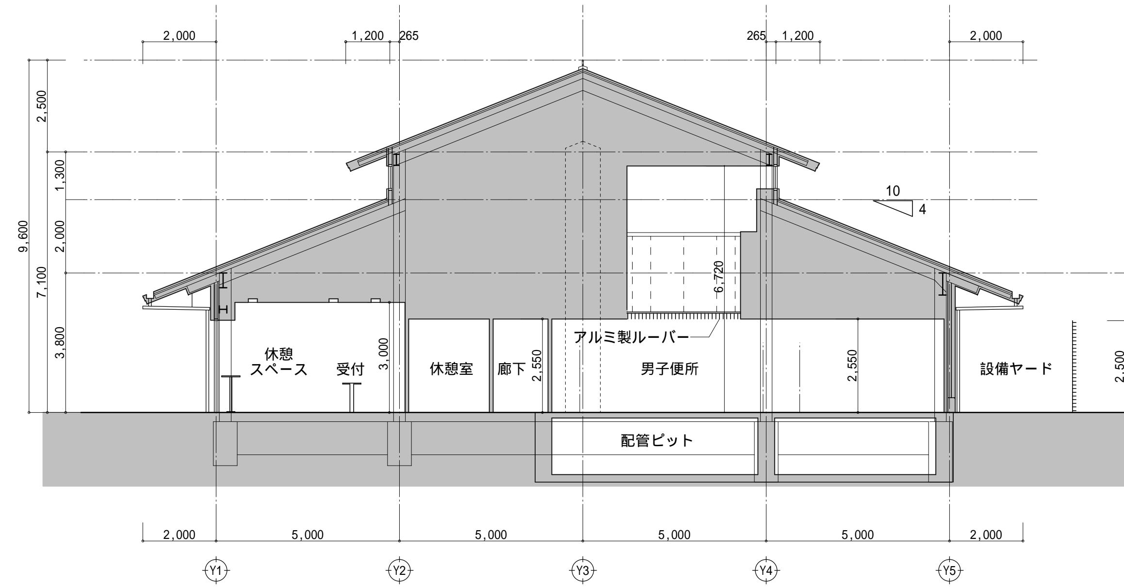
X 方向断面図 1
