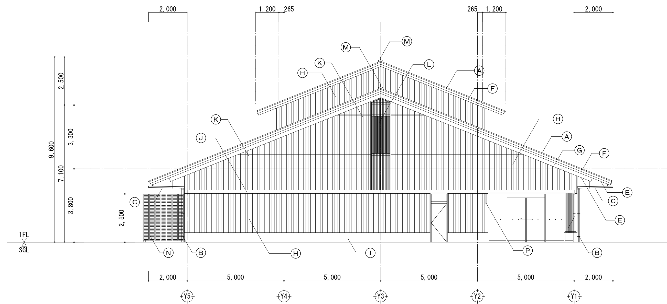
西側立面図
