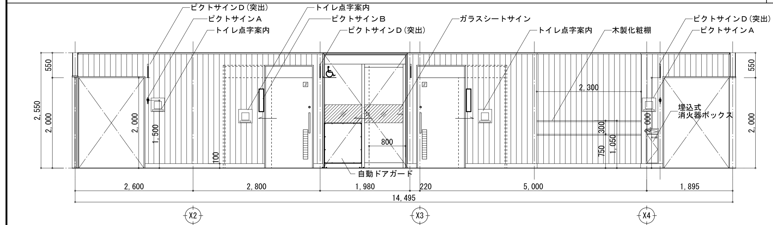
廊下 A面
