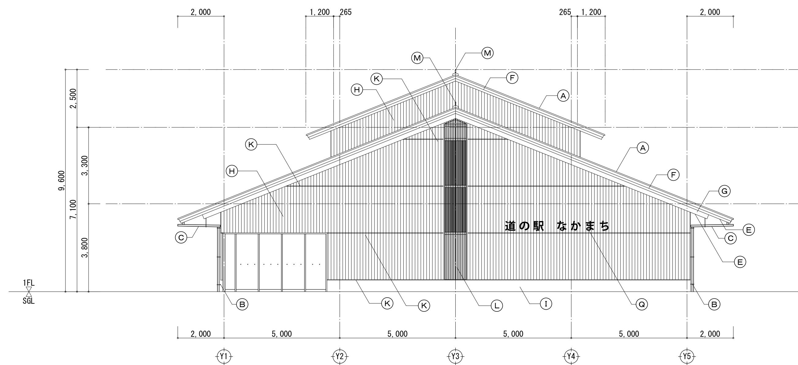
東側立面図
