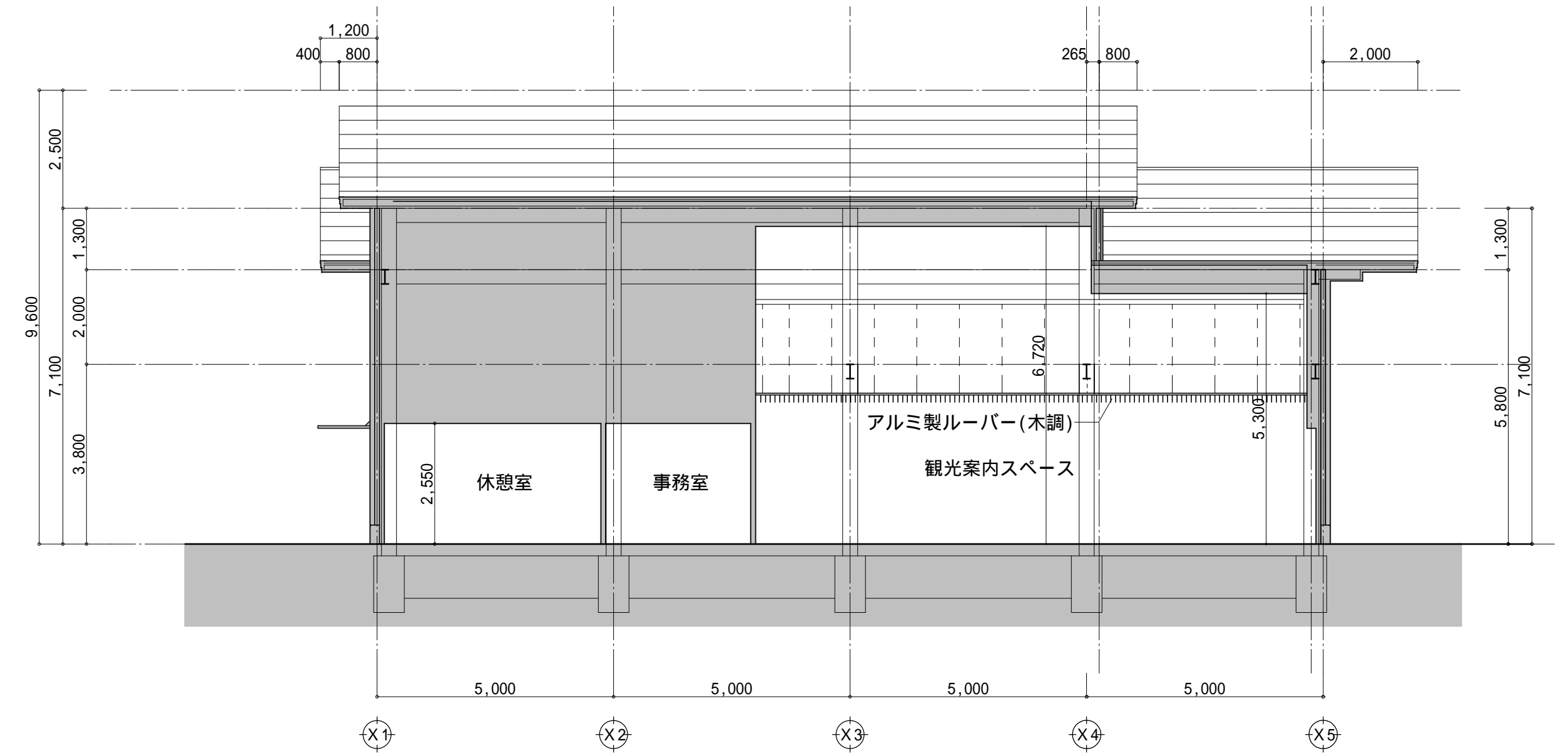
Y 方向断面図
