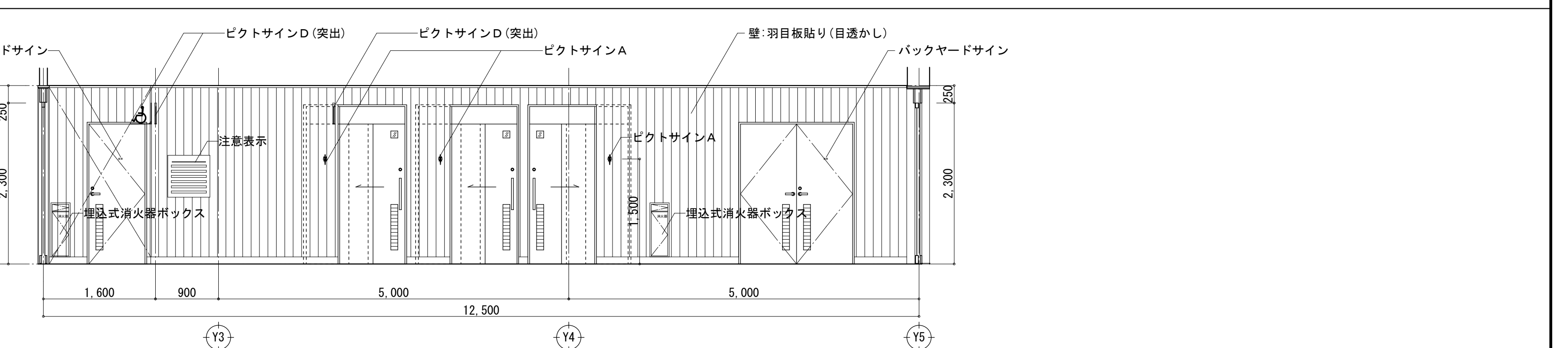
廊下 D面
