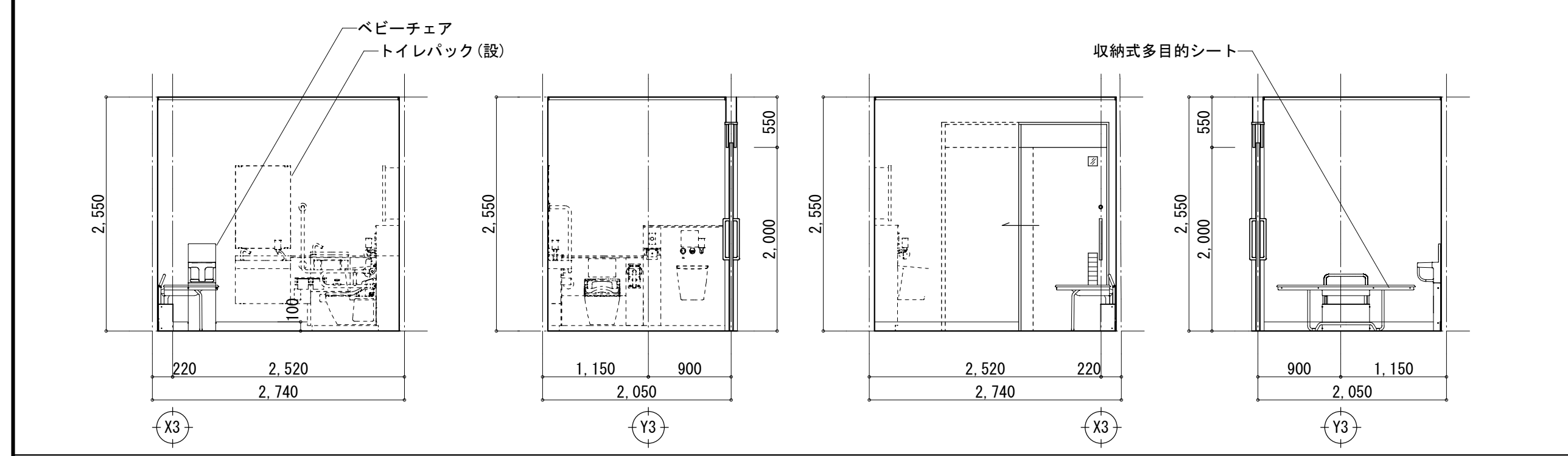
バリアフリートイレ2 A面 B面 C面 D面 授乳室1 A面 B面 C面 D面
