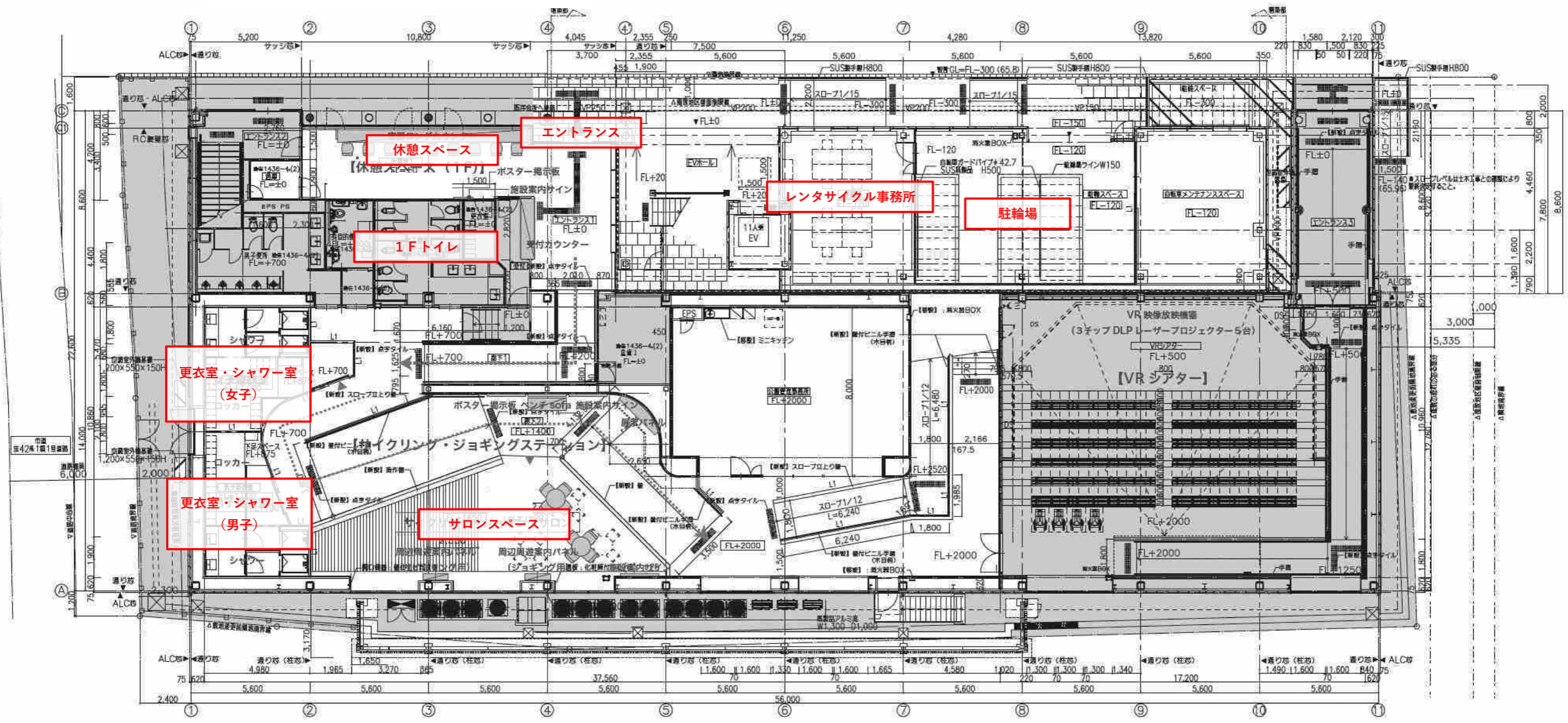
1階平面図
