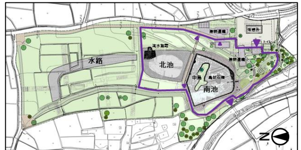
飛鳥京跡苑池(南池)基本設計図
