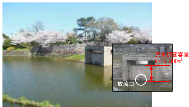
図 7-3 ため池の治水利用 (鰻堀池・大和郡山市)
