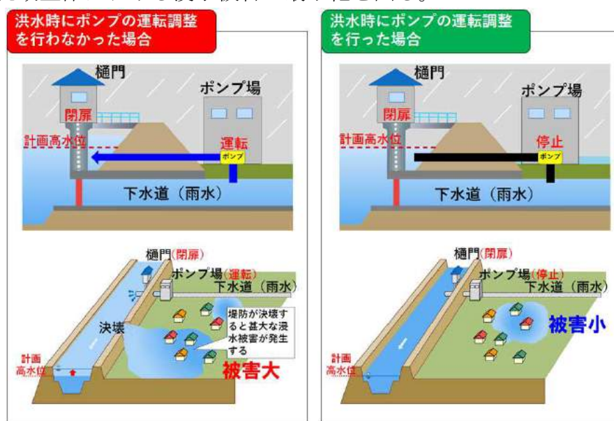
図9 内水排除ポンプの運転イメージ
