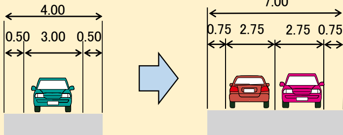
◆標準断面図 (単位:m)
