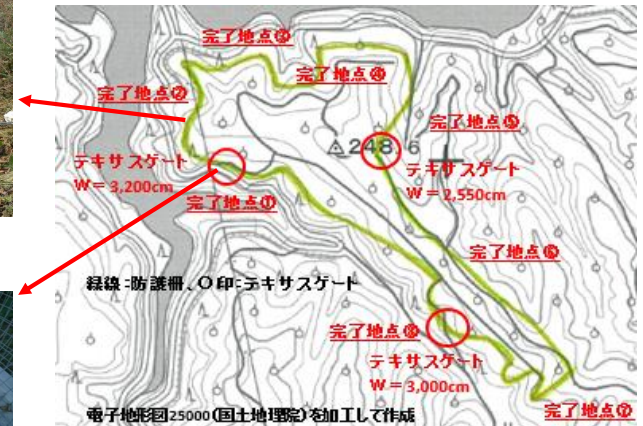
共同作業による防護柵(ワイヤーメッシュ柵)の設置
