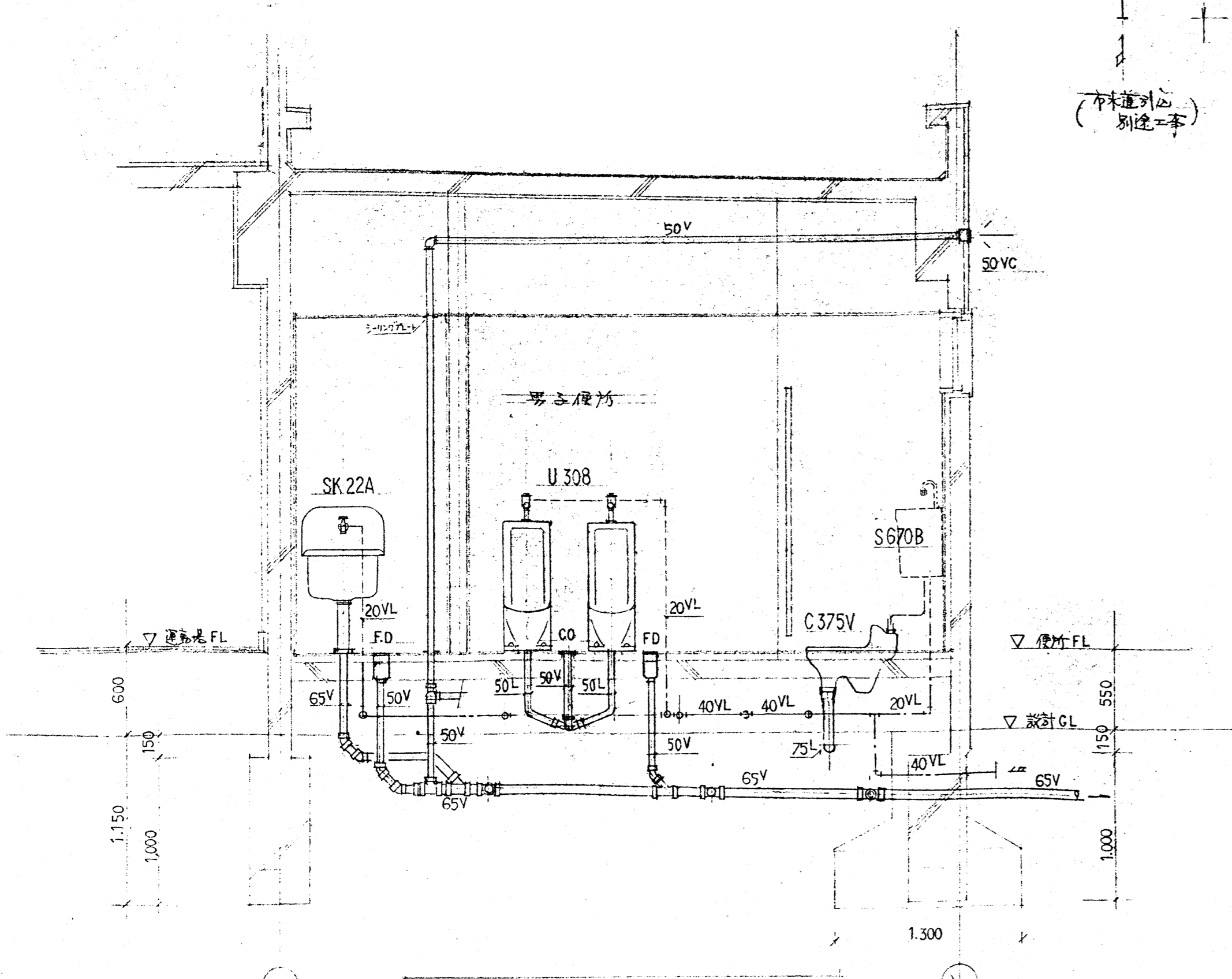
平面詳細図 1/30
