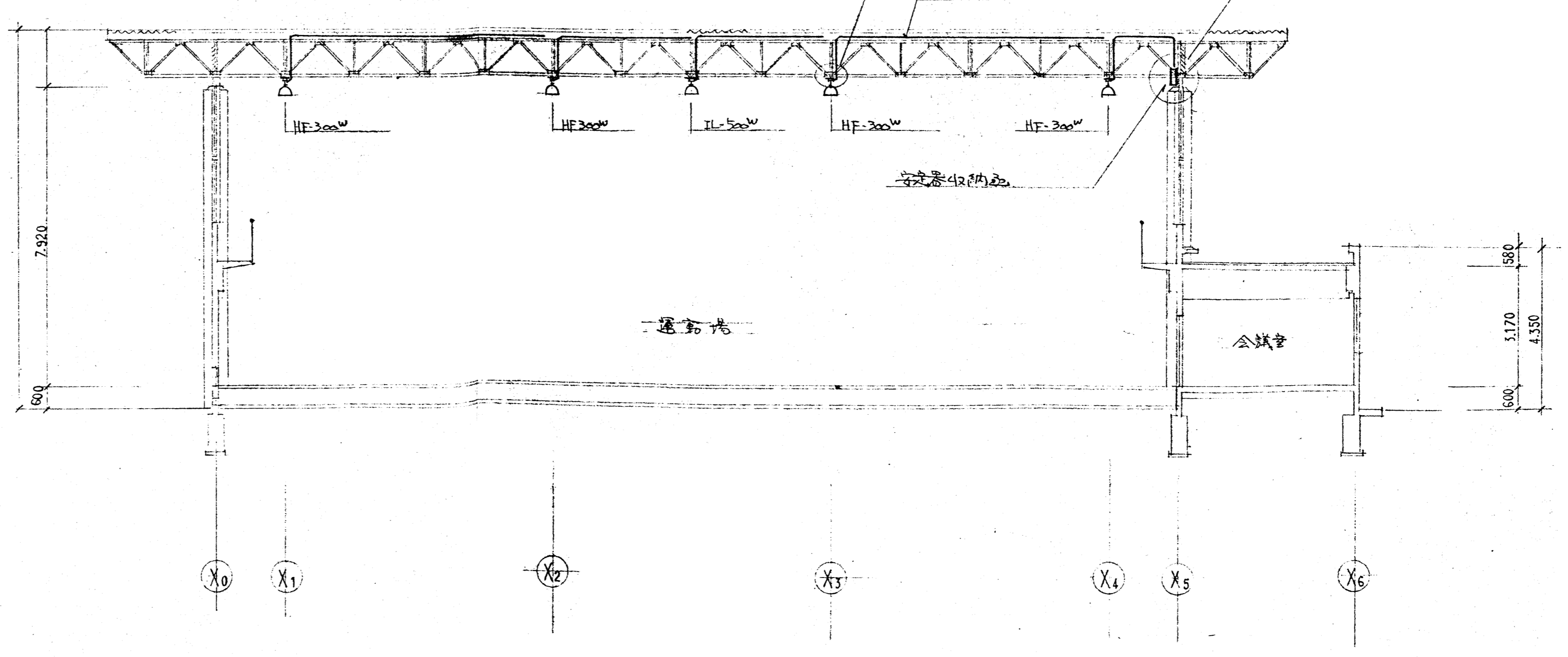
断面図 1/100
