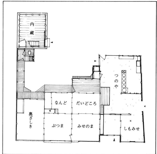
旧臼井家住宅現状平面図
