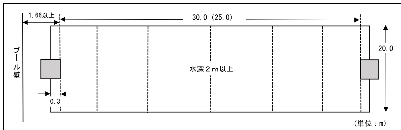
【図 3】 水球用プール
