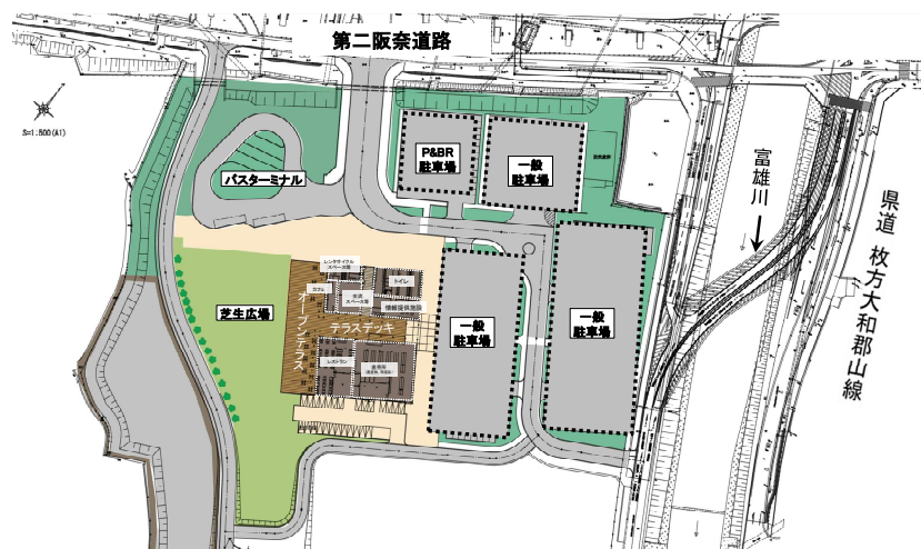
図 2.5 中町「道の駅」整備イメージ
