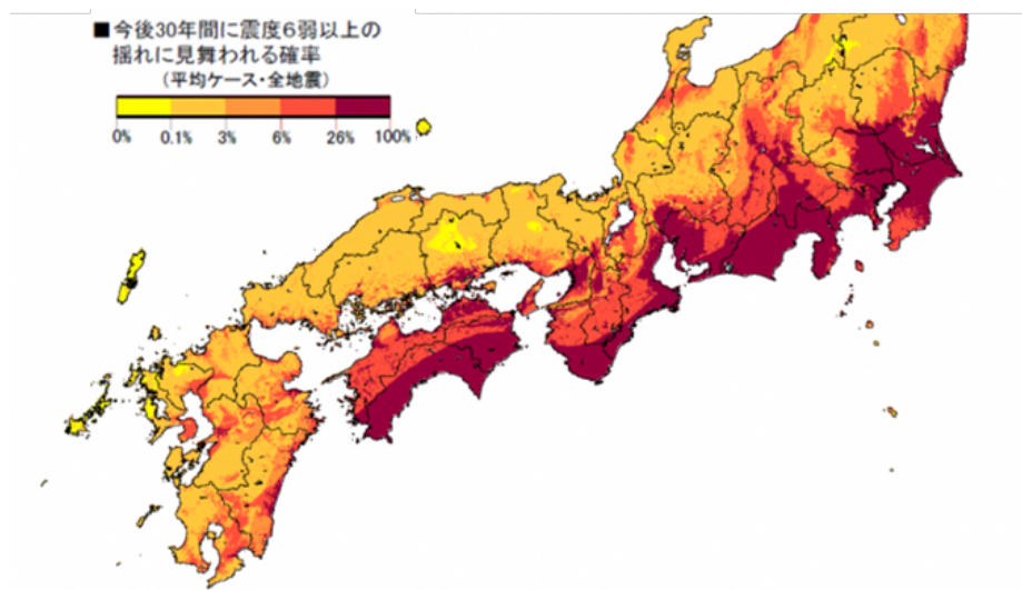
図 1.19 今後 30 年間に震度 6 弱以上の揺れに見舞われる確率 (平均ケース・全地震)
