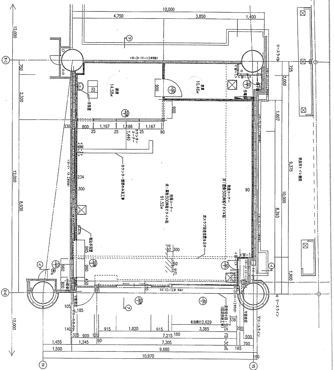
平面詳細図
