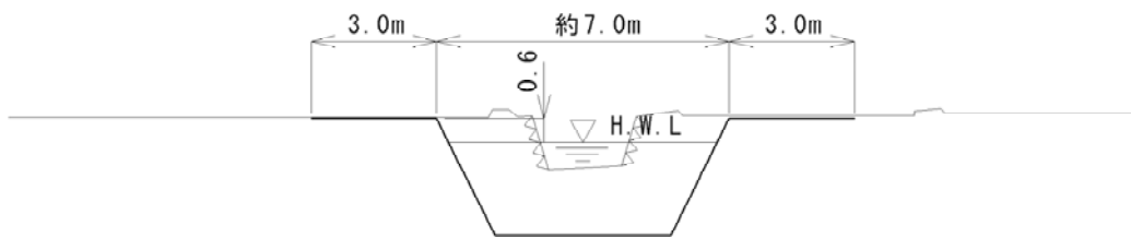
図(8)-2 高田東高校付近の横断面図*
