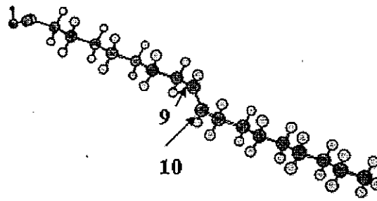
エライジン酸 C18:1 (9- trans ) 融点 46.5℃
