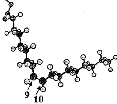
オレイン酸 C18:1 (9- cis ) 融点 13.4℃
