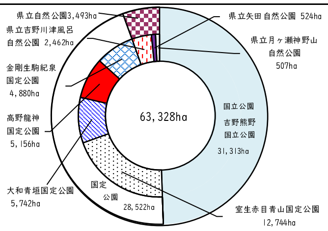
奈良県の自然公園面積一覧
