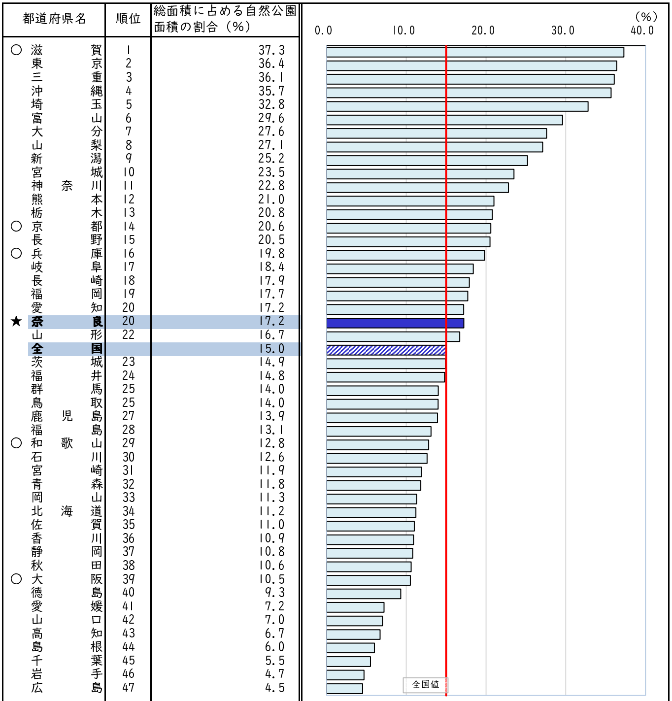
奈良県の自然公園面積一覧
