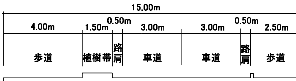
標準横断面
