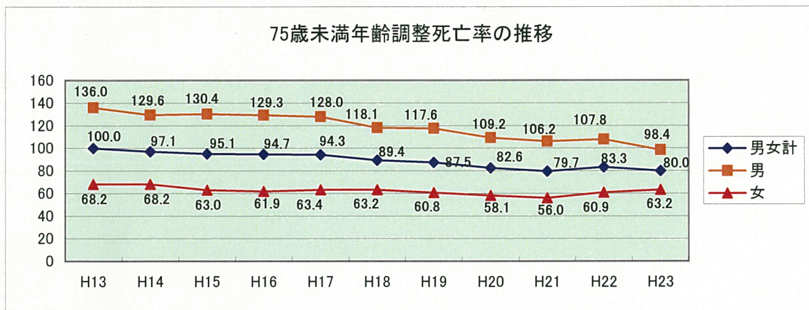
【表3】75歳未満年齢調整死亡率の増加(H22年度との比較)
