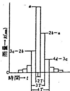
図2-1 ハイトグラフのつくり方
