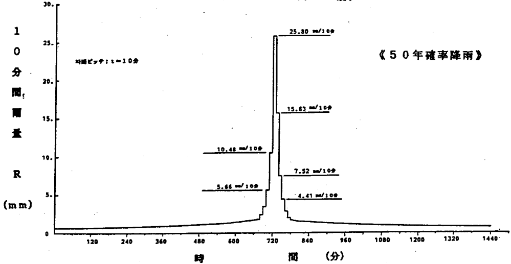
図2-2 中央集中型確率降雨波形 表2-2 奈良県確率降雨強度式
