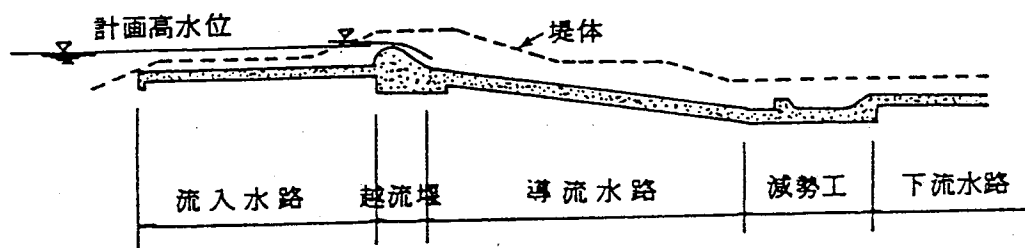
図 3 - 4 ダム式の余水吐の一般図
