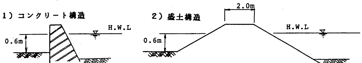
図3-1 小堤・小掘込式
