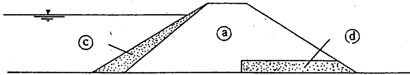
(1) 均一形ダム
